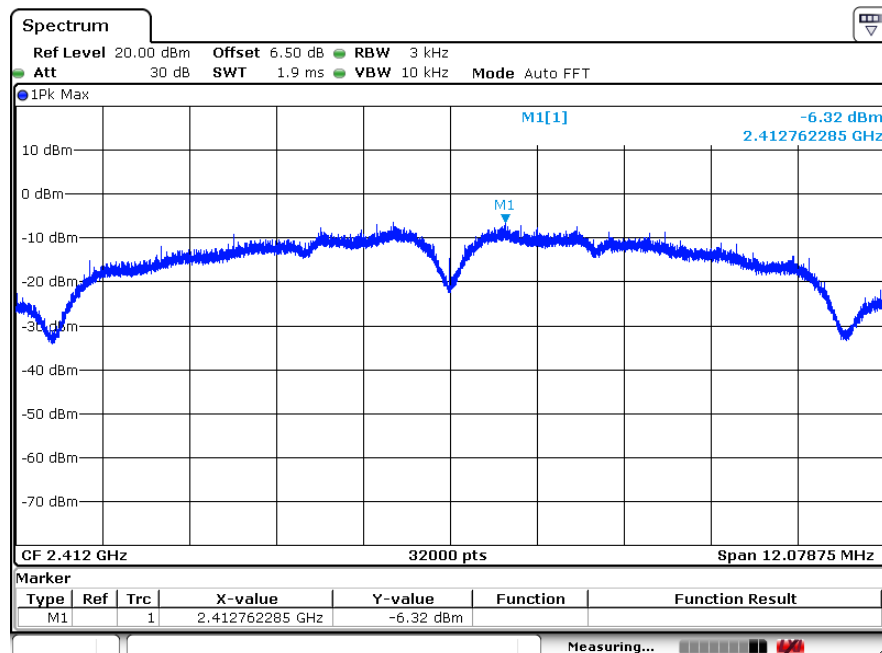
802.11 B Mode CH1
