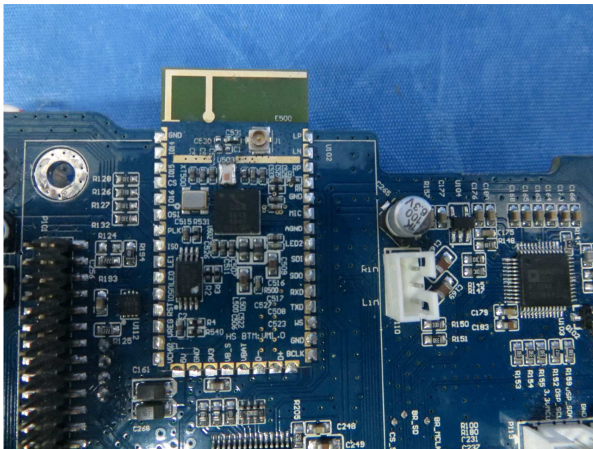
BT module
