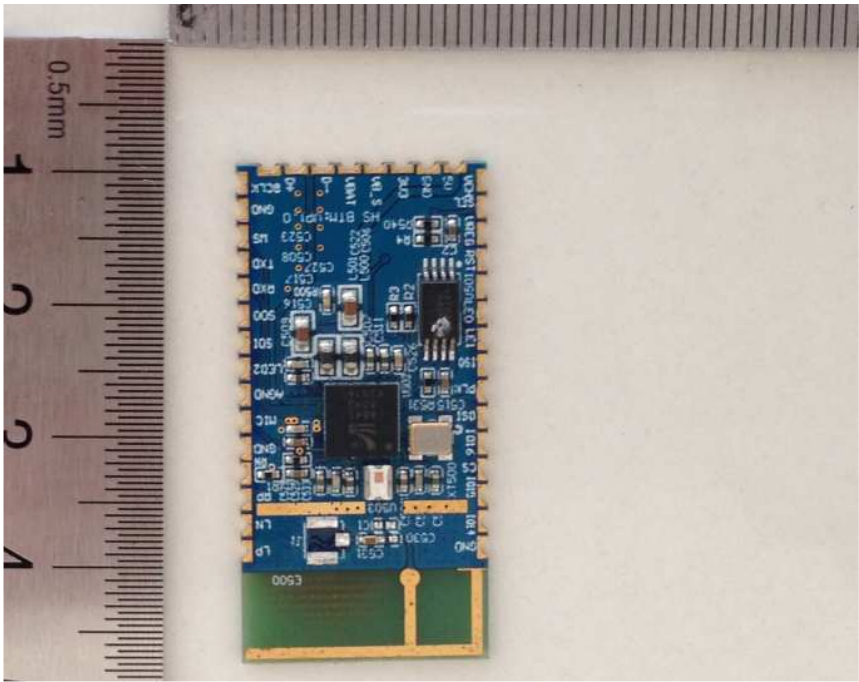
BT module
