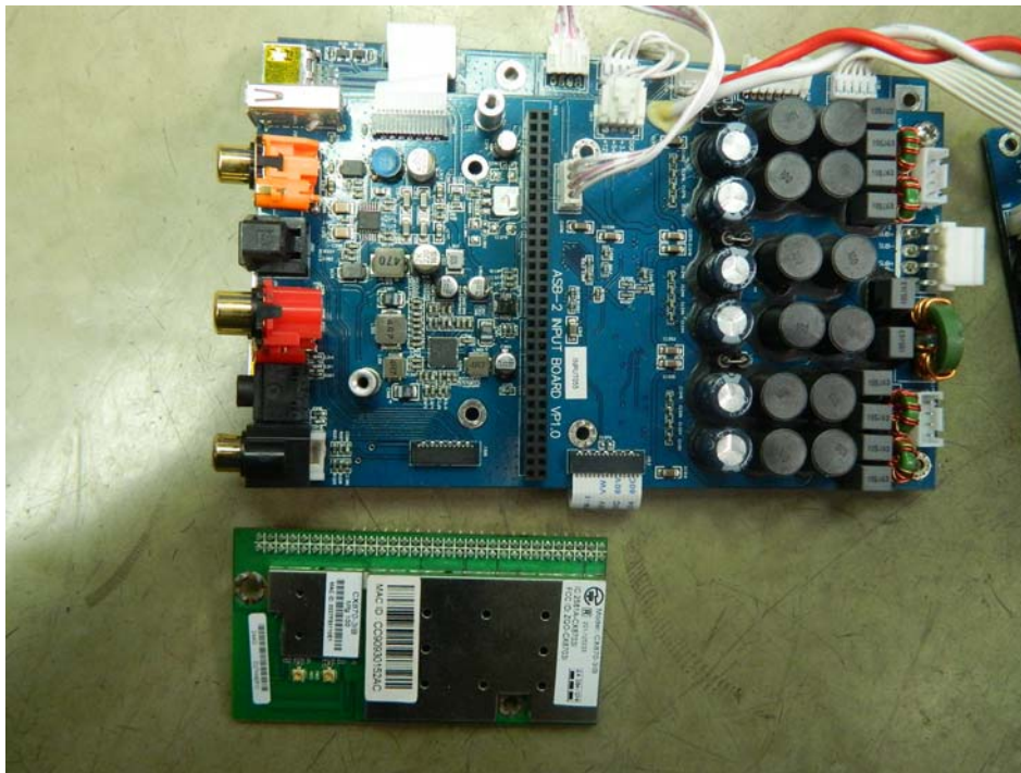
RF module
