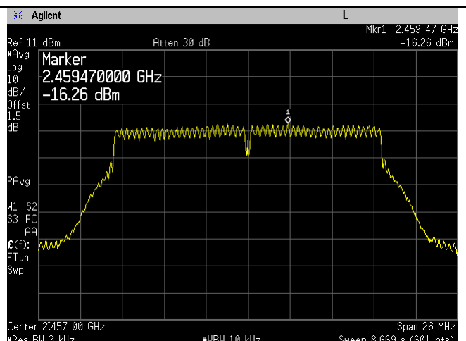
802.11g - 10 CH 2457
