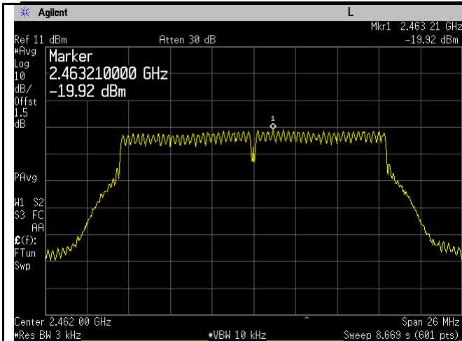
802.11g - 11 CH 2462
