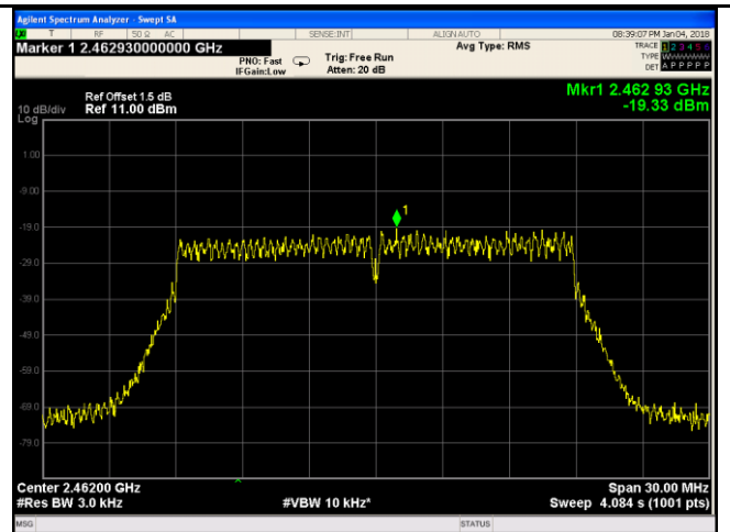
802.11n20 - 11 CH 2462
