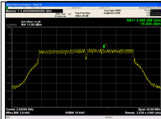
802.11g - 11 CH 2462
