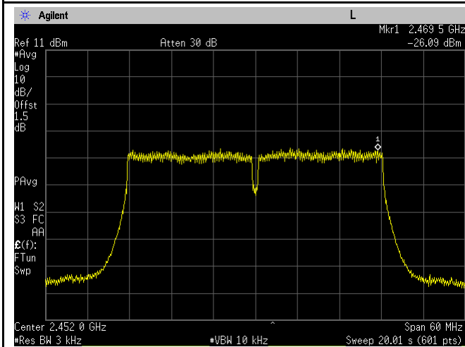
802.11n40 - 9 CH 2452
