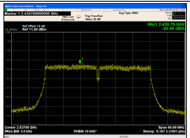
802.11n40 - 6 CH 2437
