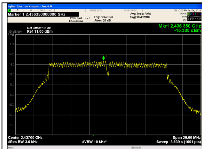
802.11g - 6 CH 2437
