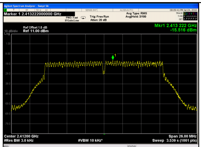
802.11g - 1 CH 2412
