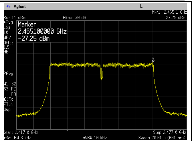
802.11n40 - 8 CH 2447
