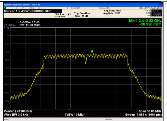
802.11n20 - 1 CH 2412
