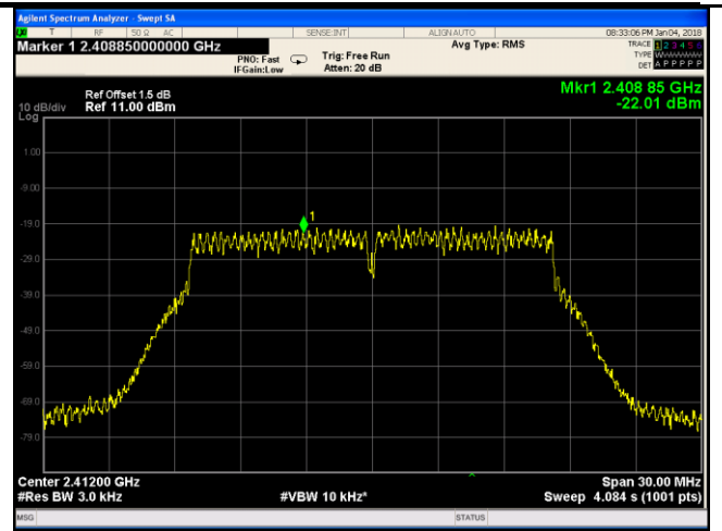
802.11n20 - 1 CH 2412
