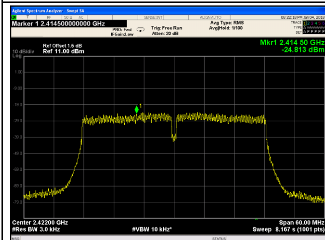
802.11n40 - 3 CH 2422
