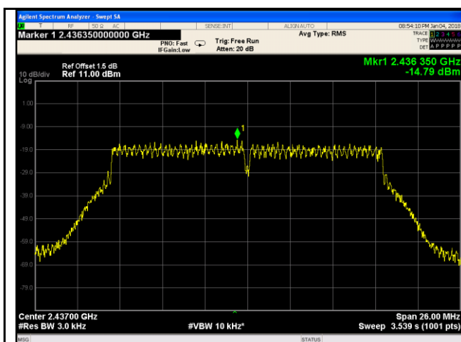
802.11g - 6 CH 2437
