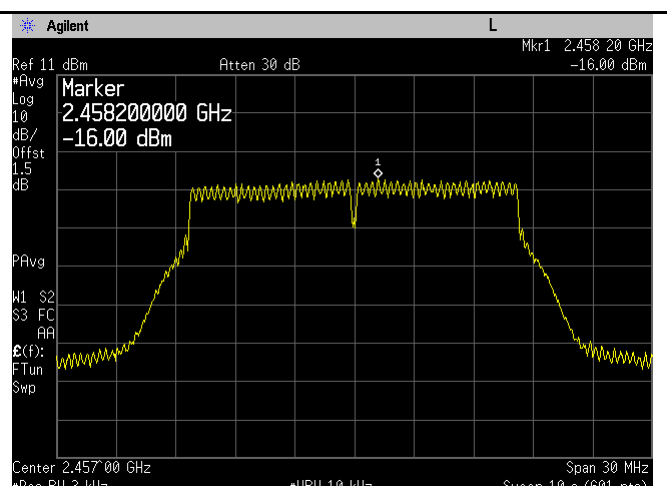
802.11g - 10 CH 2457
