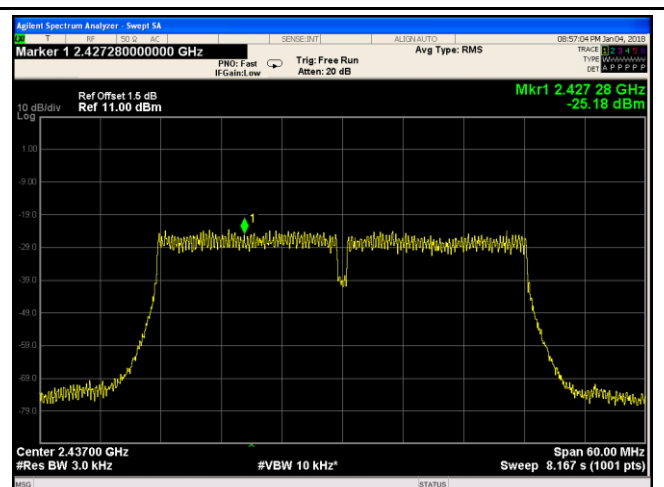
802.11n40 - 6 CH 2437
