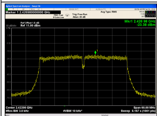
802.11n40 - 3 CH 2422
