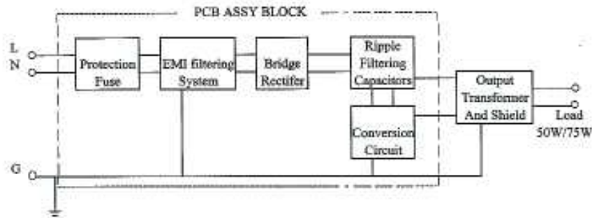
50W/75W Diagram
