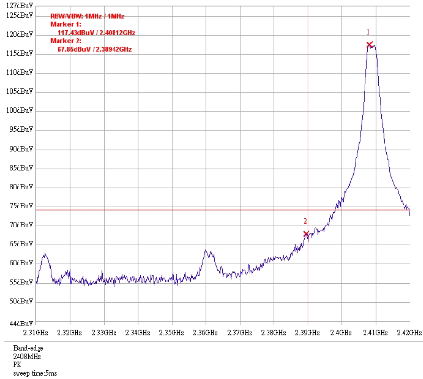
Band edge @ channel 1 PK
