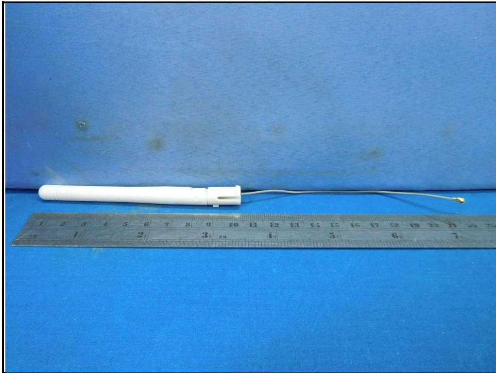
Antenna: VM2506TX(202-000521-00)
