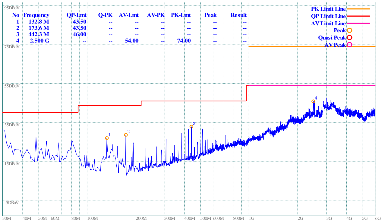
(Plot A: 30MHz – 6GHz, Test Antenna Vertical)
