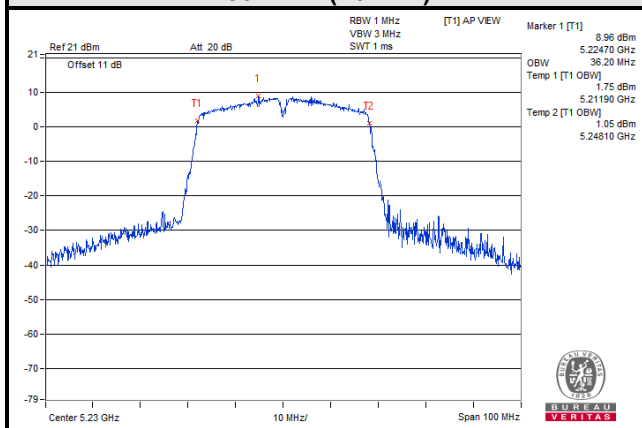
802.11n (40MHz)
