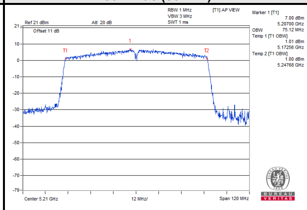
802.11ac (80MHz)
