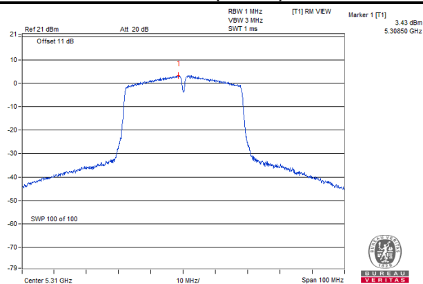
802.11ac (40MHz)
