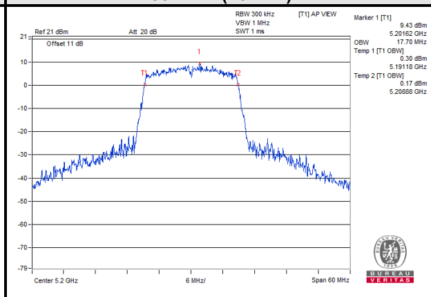
802.11ac (20MHz)
