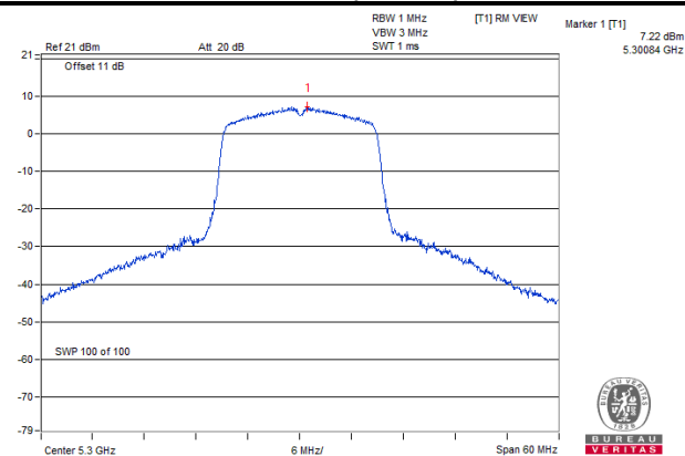
802.11ac (20MHz)
