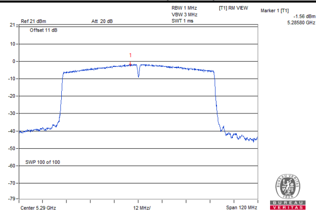
802.11ac (80MHz)
