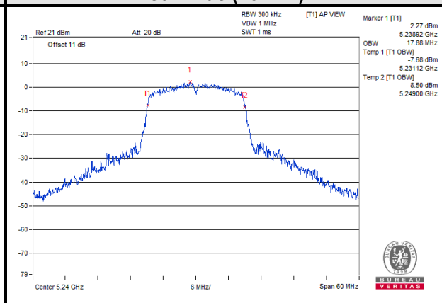
802.11ac (20MHz)
