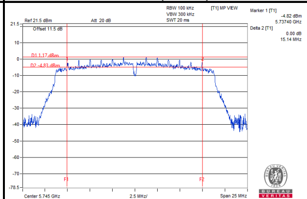
802.11ac (20MHz)
