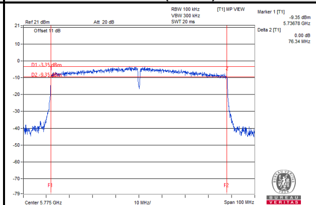
802.11ac (80MHz)
