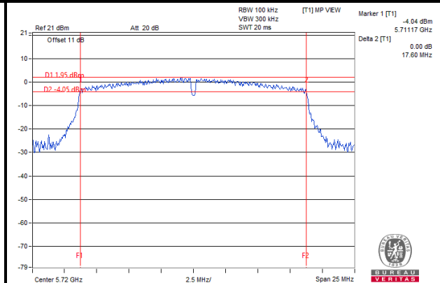
802.11ac (20MHz)
