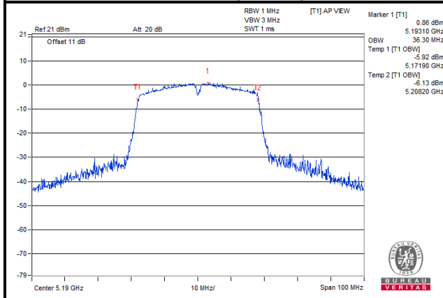
802.11ac (40MHz)
