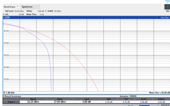
Band25-20MHz-16QAM-26590-1RB#0
