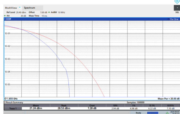
Band25-10MHz-16QAM-26340-50RB#0
