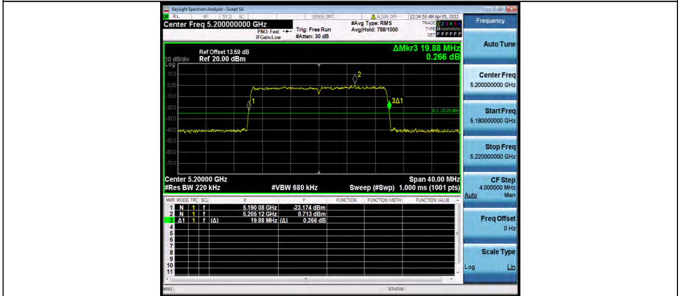
11AX20MIMO_Ant1_5200_26Tone_RU0
