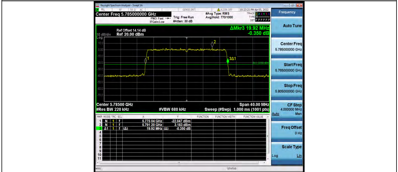
11AX20MIMO_Ant1_5785_26Tone_RU0
