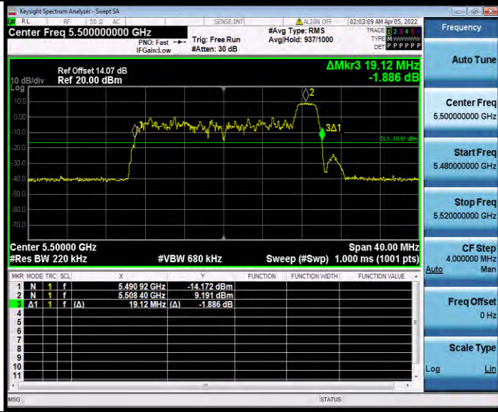
11AX20MIMO_Ant0_5500_242Tone_RU61
