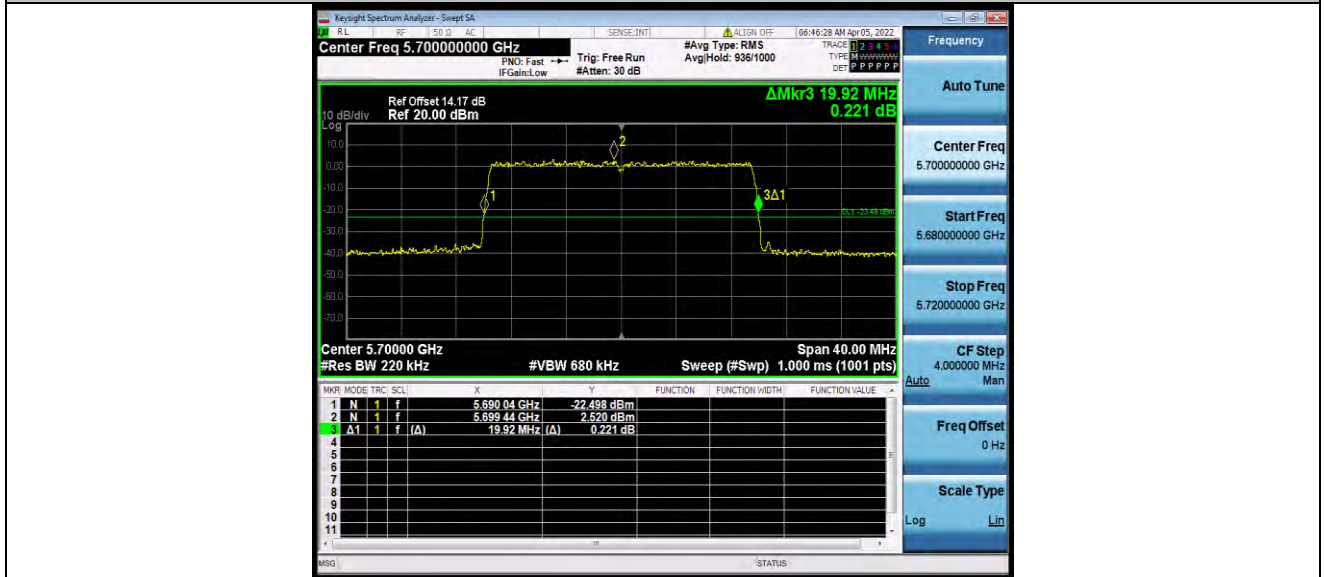
11AX20MIMO_Ant1_5700_26Tone_RU0
