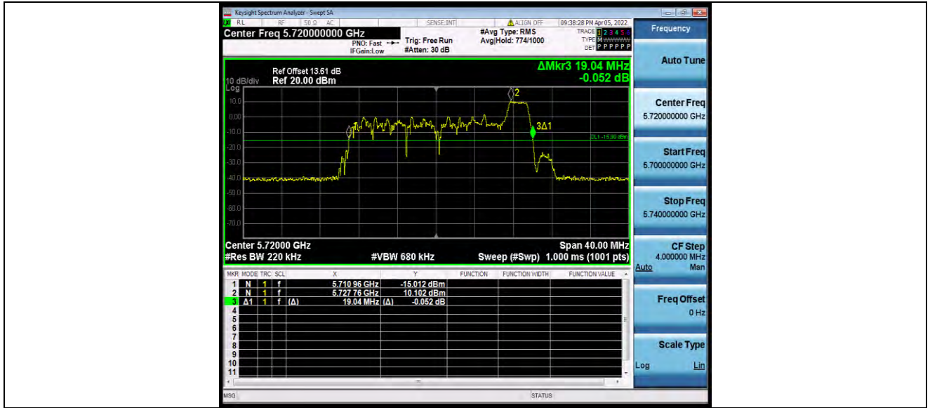
11AX20MIMO_Ant1_5720_242Tone_RU61
