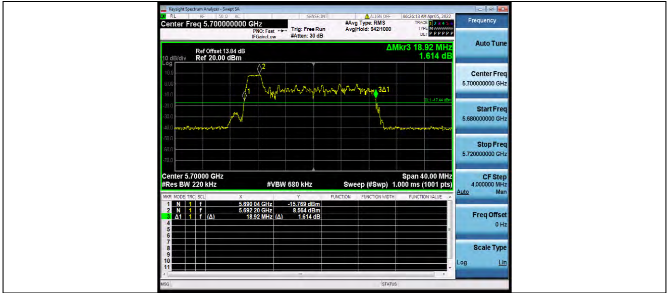
11AX20MIMO_Ant1_5700_26Tone_RU4
