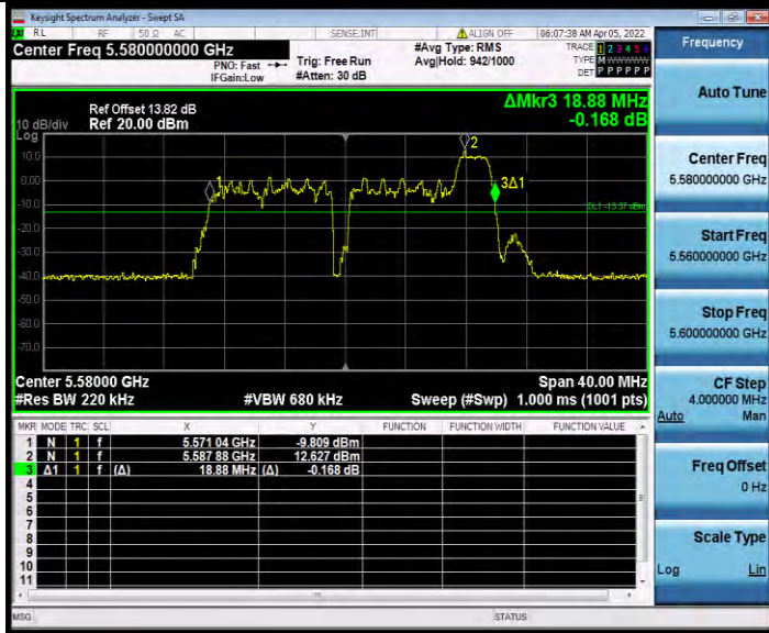
11AX20MIMO_Ant1_5580_242Tone_RU61
