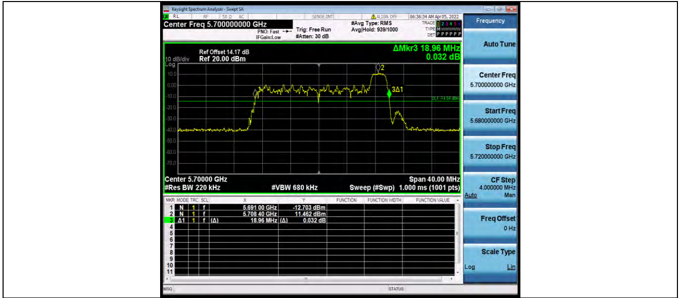
11AX20MIMO_Ant0_5700_242Tone_RU61
