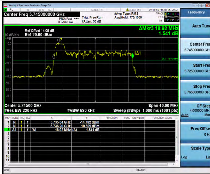
11AX20MIMO_Ant0_5745_26Tone_RU4
