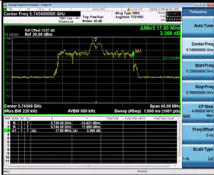
11AX20MIMO_Ant1_5745_26Tone_RU8
