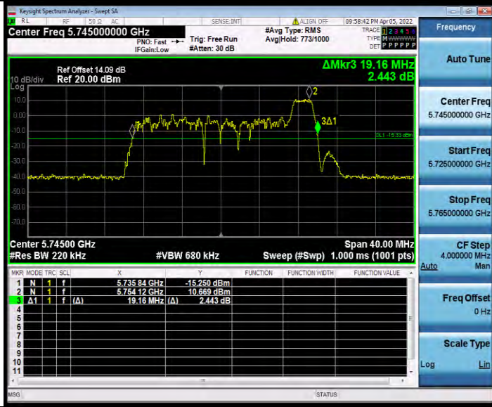
11AX20MIMO_Ant0_5745_242Tone_RU61
