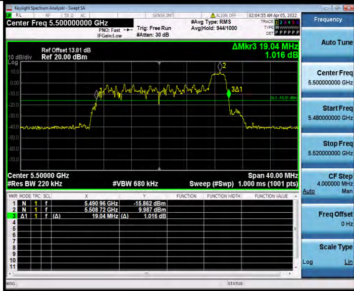
11AX20MIMO_Ant1_5500_242Tone_RU61
