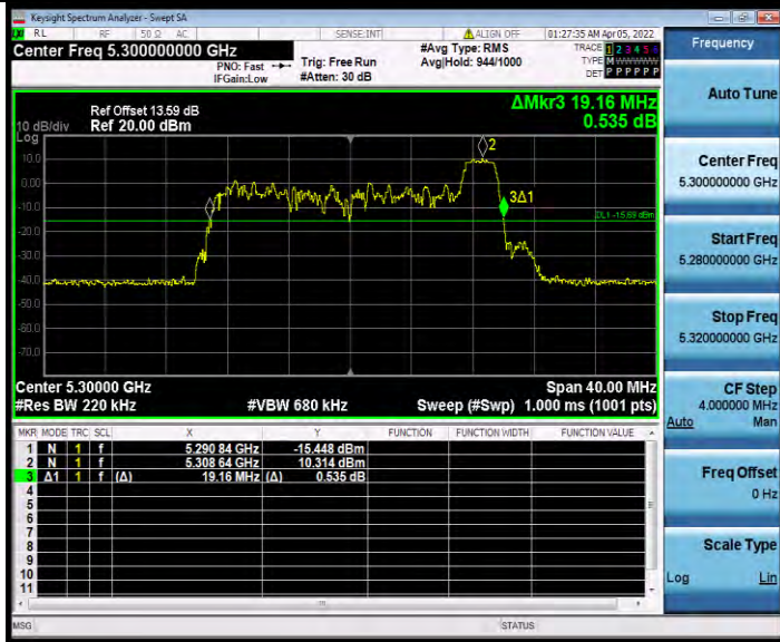
11AX20MIMO_Ant1_5300_242Tone_RU61
