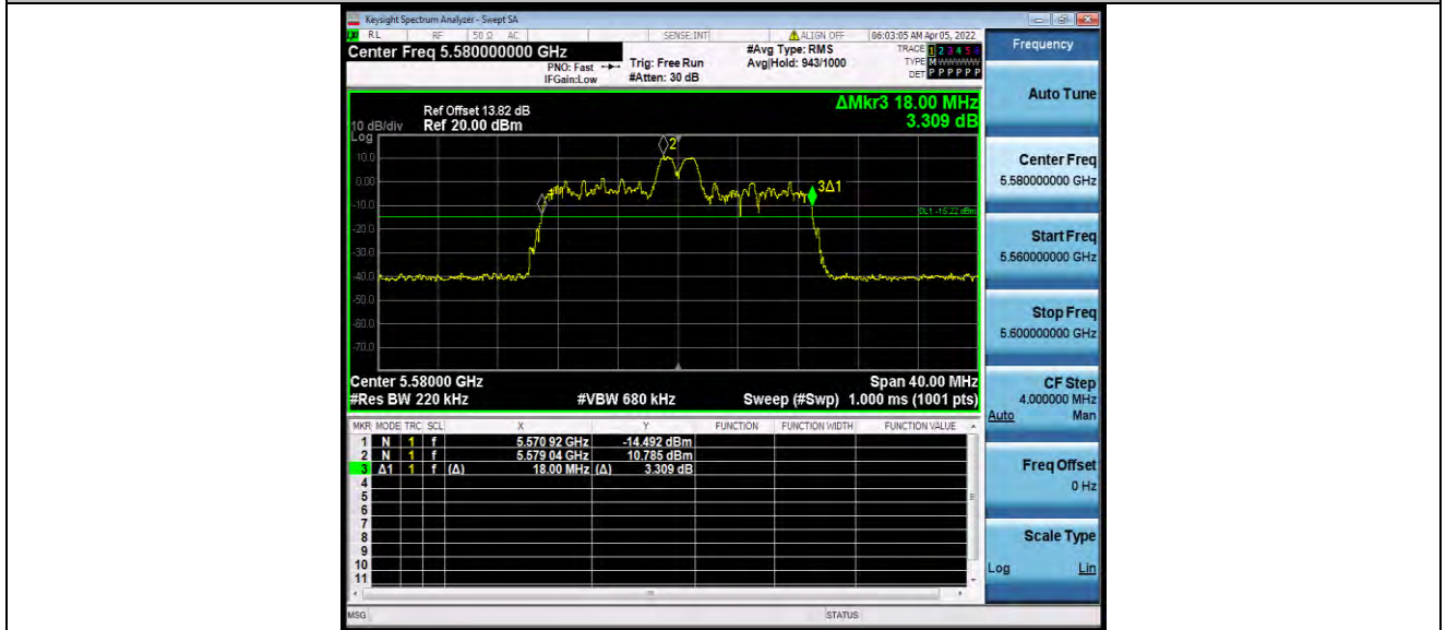
11AX20MIMO_Ant1_5580_26Tone_RU8
