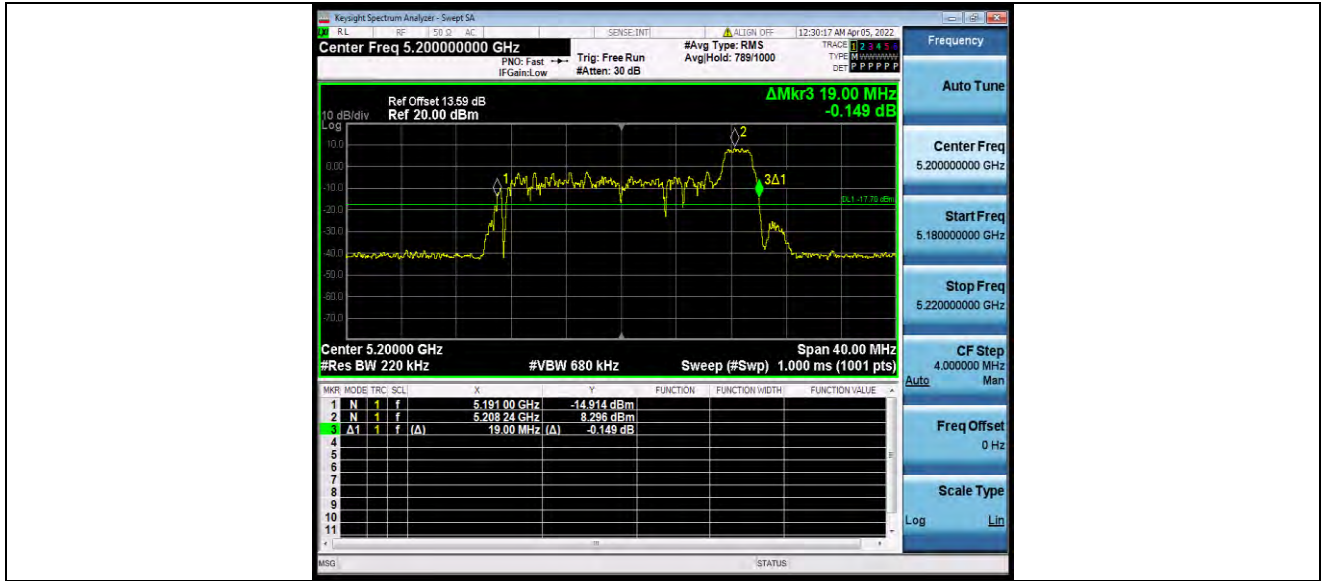
11AX20MIMO_Ant0_5200_242Tone_RU61
