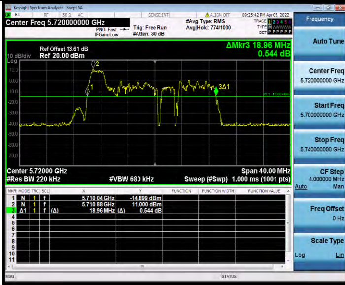
11AX20MIMO_Ant1_5720_26Tone_RU4
