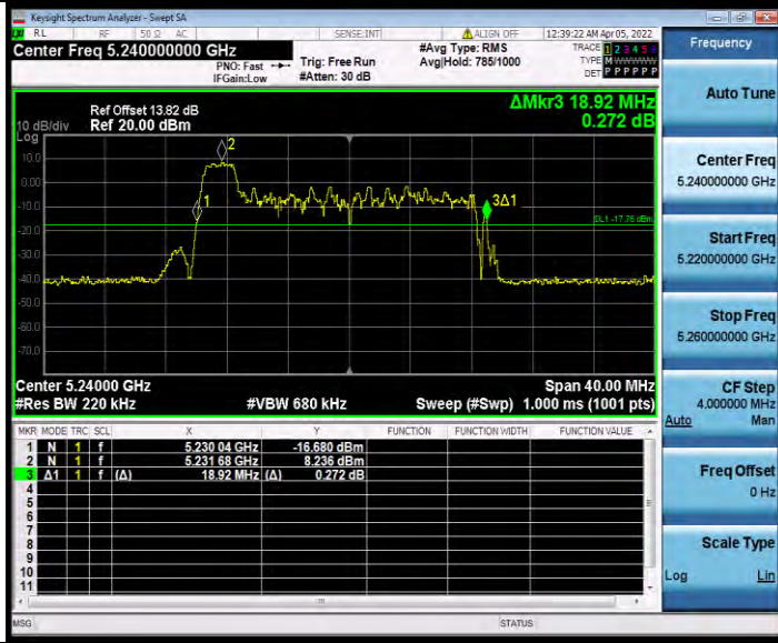
11AX20MIMO_Ant0_5240_26Tone_RU4
