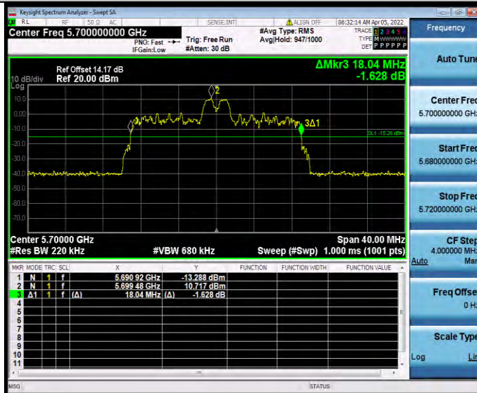
11AX20MIMO_Ant0_5700_26Tone_RU8
