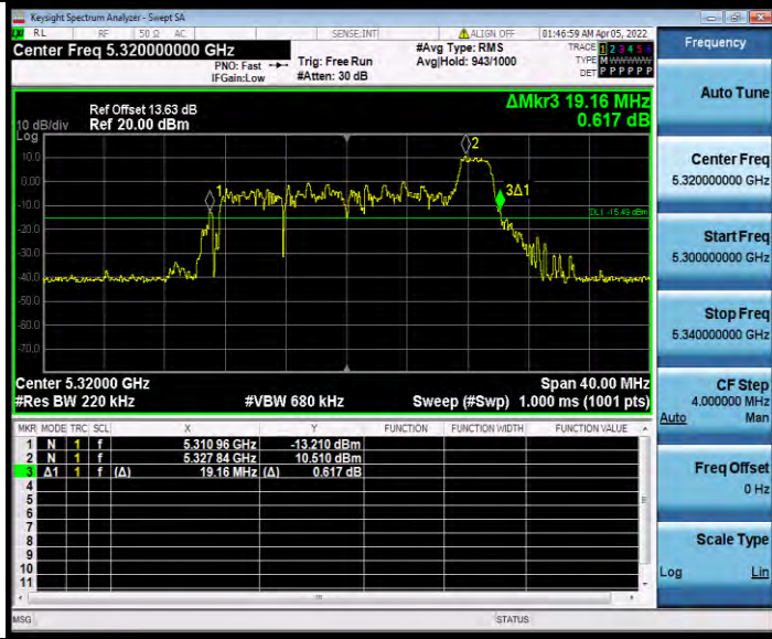
11AX20MIMO_Ant1_5320_242Tone_RU61
