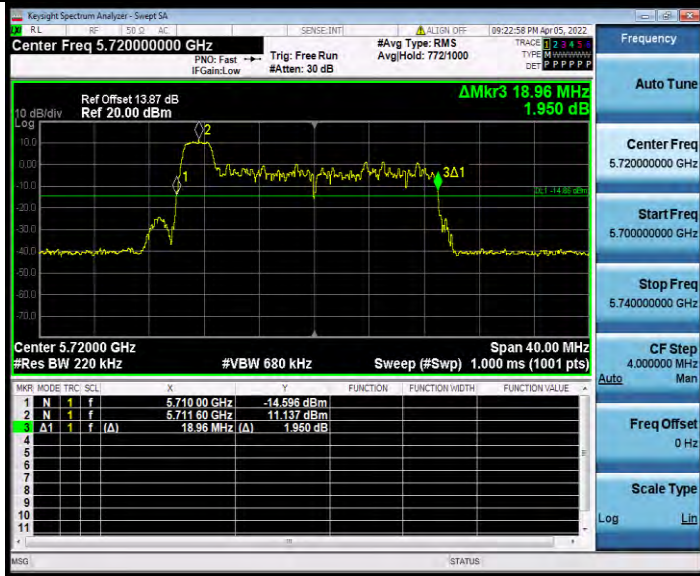
11AX20MIMO_Ant0_5720_26Tone_RU4
