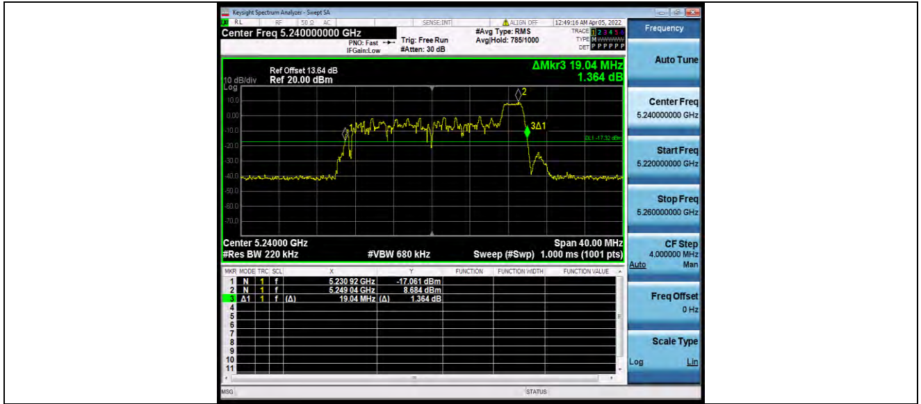
11AX20MIMO_Ant1_5240_242Tone_RU61
