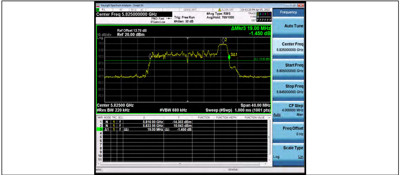
11AX20MIMO_Ant1_5825_242Tone_RU61
