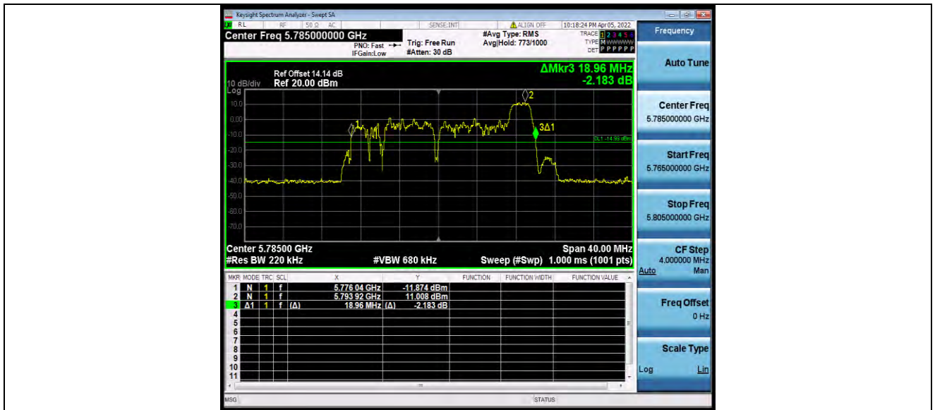
11AX20MIMO_Ant0_5785_242Tone_RU61
