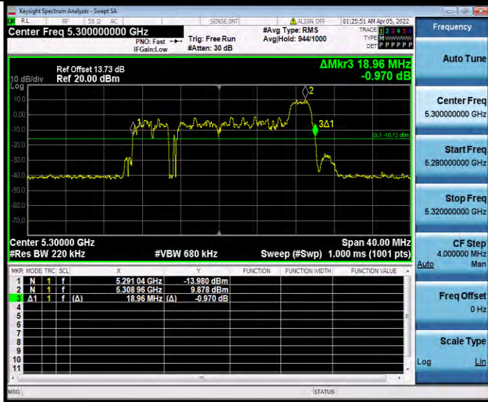
11AX20MIMO_Ant0_5300_242Tone_RU61
