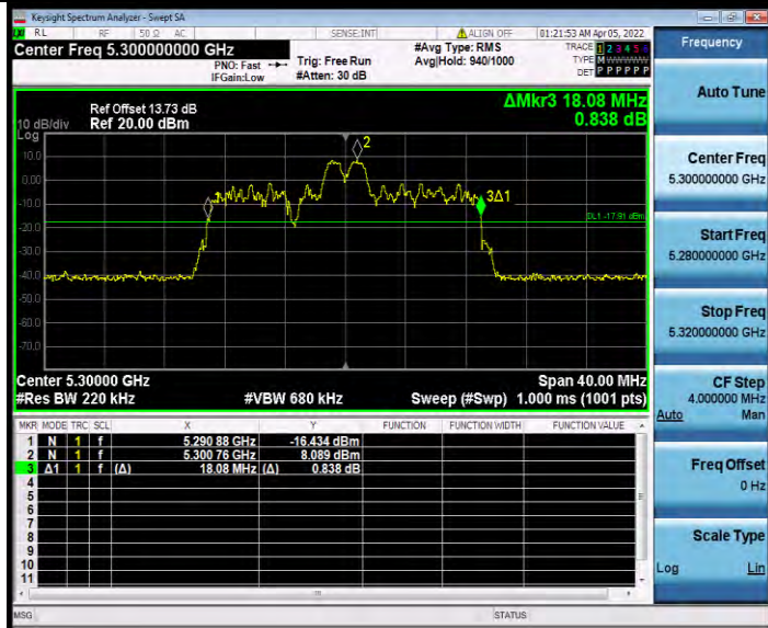
11AX20MIMO_Ant0_5300_26Tone_RU8
