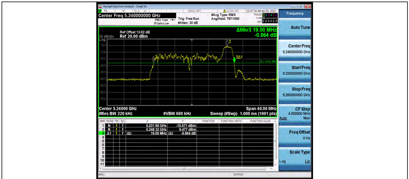
11AX20MIMO_Ant0_5240_242Tone_RU61
