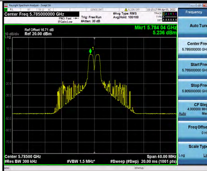
11AX20MIMO_Ant0_5785_26Tone_RU8
