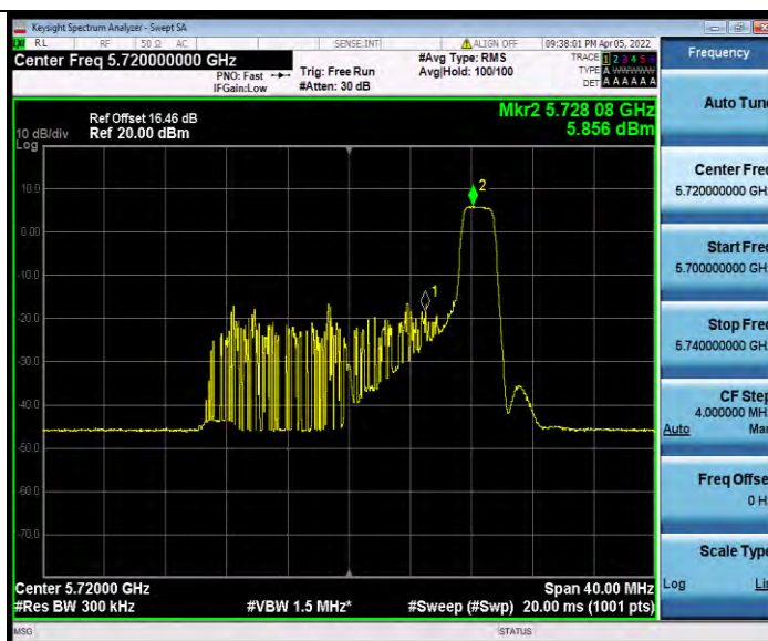
11AX20MIMO_Ant0_5720_UNII-3_242Tone_RU61
