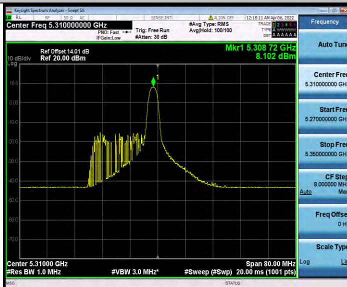
11AX40MIMO_Ant1_5310_26Tone_RU17
