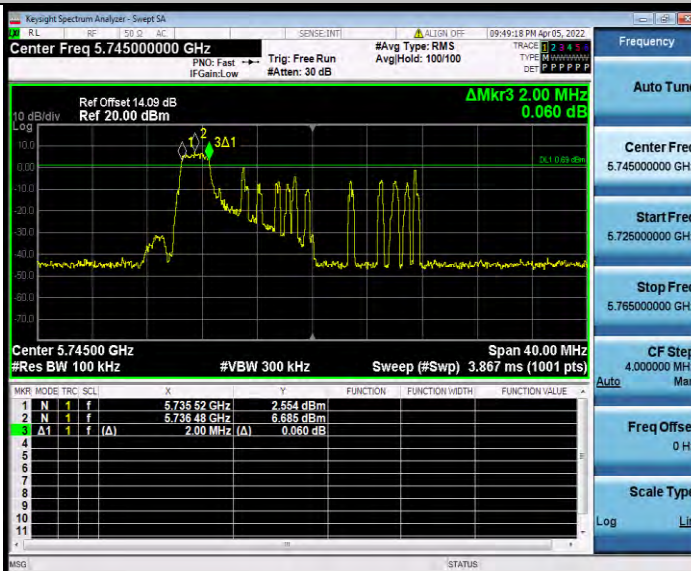
11AX20MIMO_Ant0_5745_26Tone_RU4
