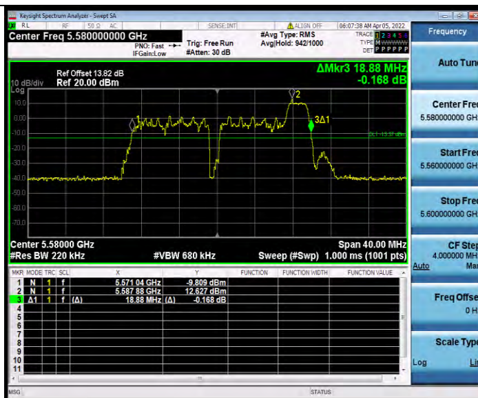
11AX20MIMO_Ant1_5580_242Tone_RU61
