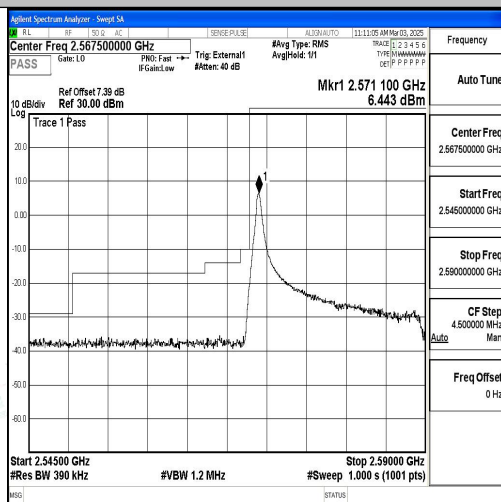
Band38 20MHz QPSK 37850 1RB#0
