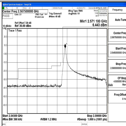
Band38 20MHz 16QAM 37850 1RB#0
