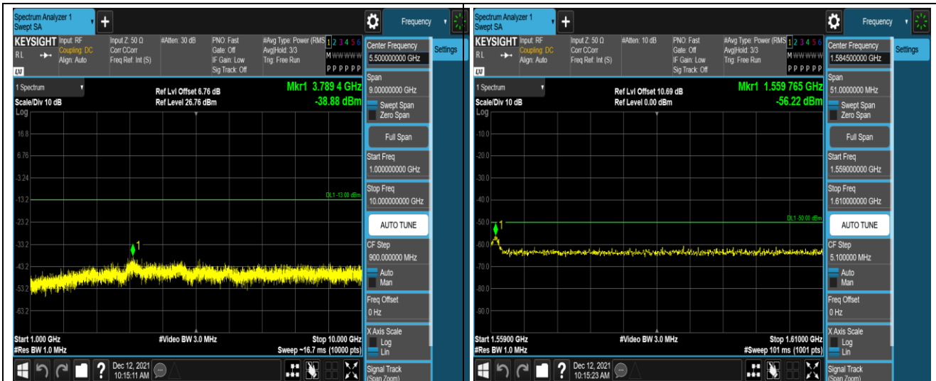
Band13-5MHz-QPSK-23230-1RB#0-Range2:1000~10000MHz
