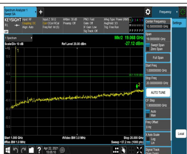
Band4-1.4MHz-QPSK-20175-1RB#0-Range2:1000~20000MHz
