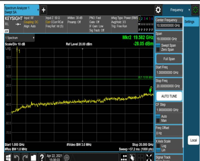
Band4-1.4MHz-QPSK-20393-1RB#0-Range2:1000~20000MHz
