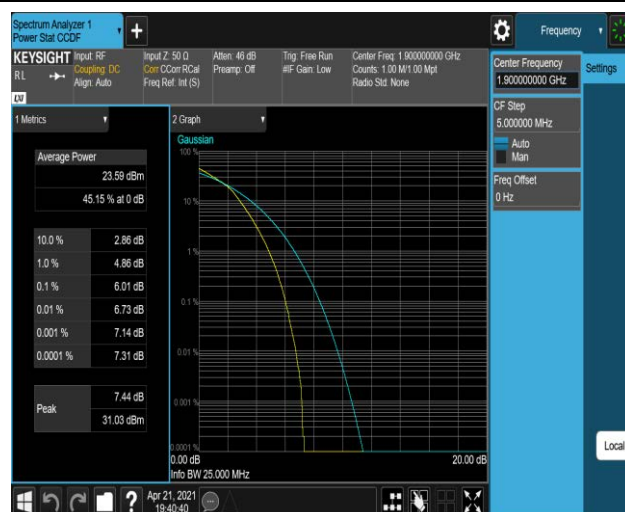
Band2-20MHz-16QAM-19100-100RB#0
