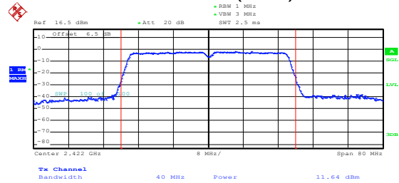
802.11n(HT40)
