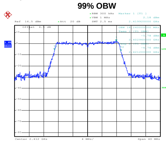
802.11n(HT20)
