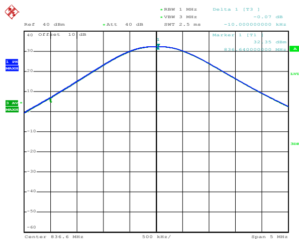
GSM 850
