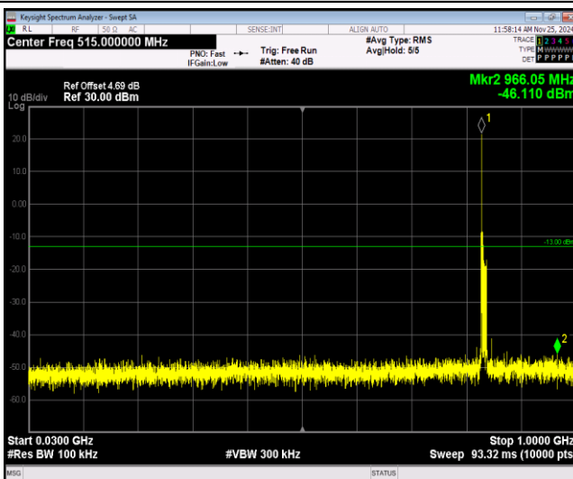
Band5-10MHz-QPSK-20600-1RB#0-Range1:30~100 0MHz
