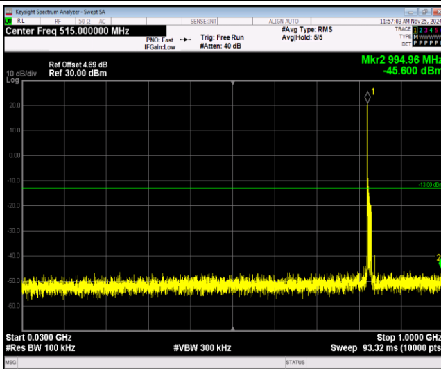
Band5-10MHz-QPSK-20525-1RB#0-Range1:30~100 0MHz
