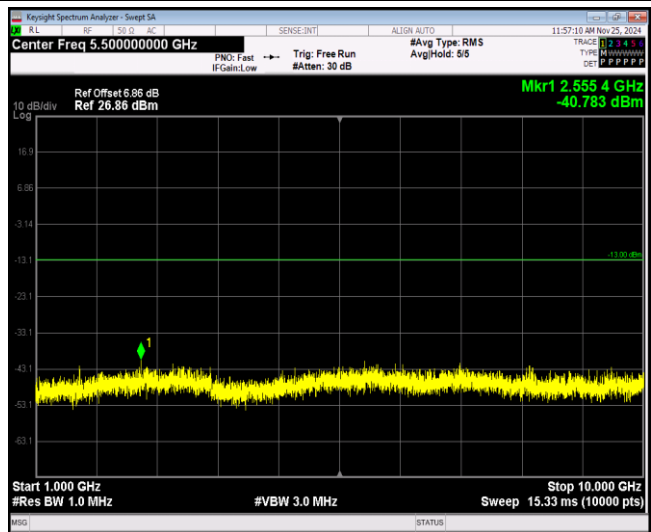
Band5-10MHz-QPSK-20525-1RB#0-Range2:1000~1 0000MHz
