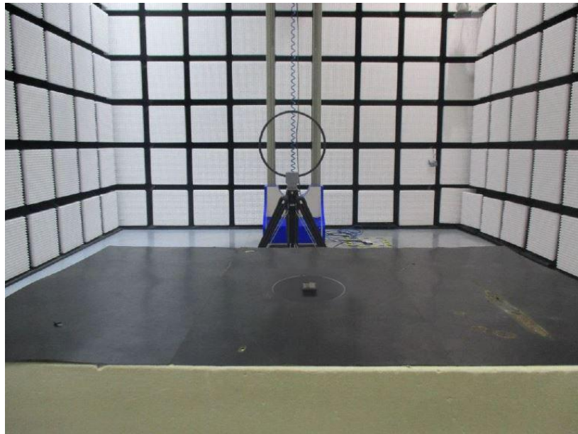
9kHz-30MHz
