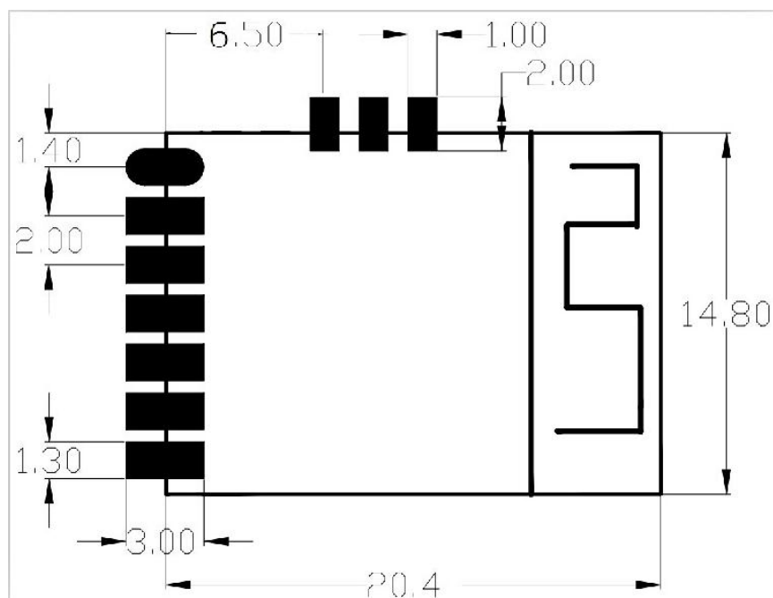
Picture3-8. Packaging(mm)
