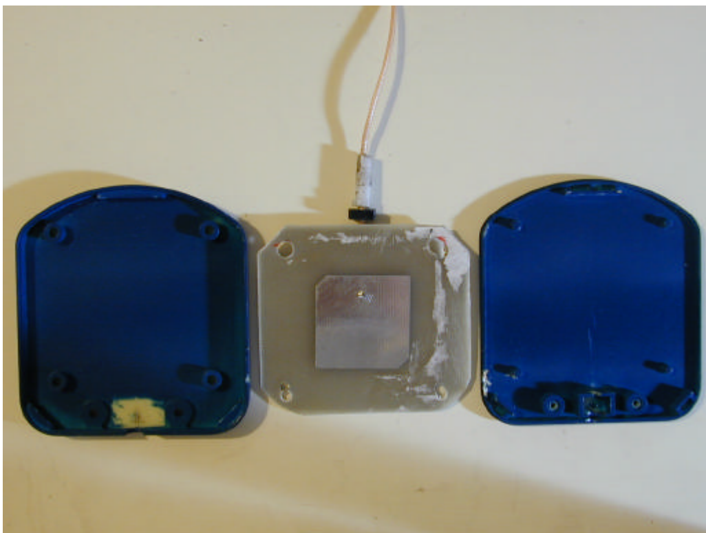
(13) EUT Photo
