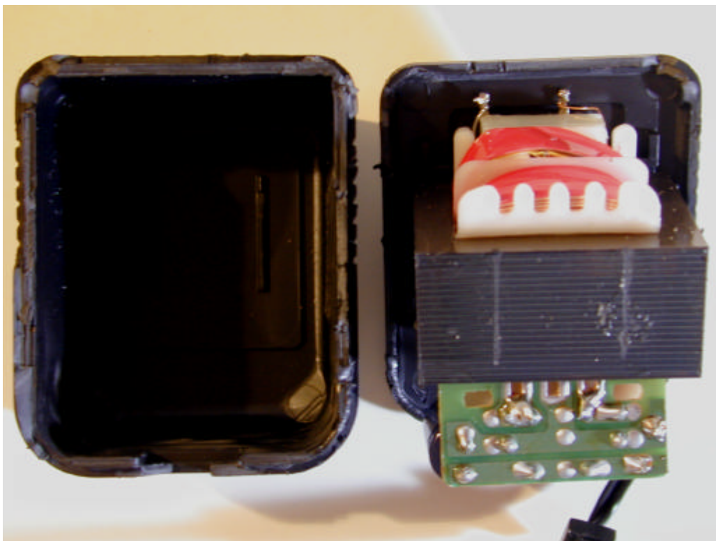
(21) EUT Photo
