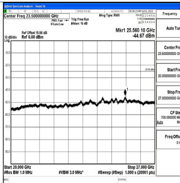
Band7_20MHz_QPSK_20850_1RB#0_20000~27000_20000~27000
