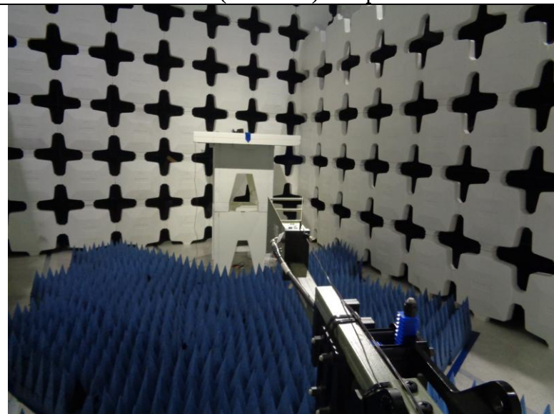
DRWG Horn (1-18GHz) Setup Overview
