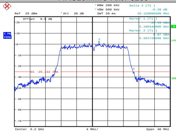
11AC20MIMO-Ant1-5200
