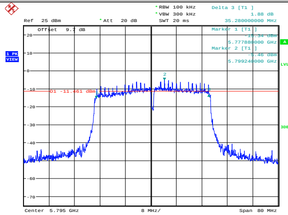
11N40MIMO-Ant1-5795
