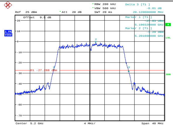
11N20MIMO-Ant2-5200
