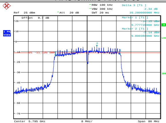
11AC40MIMO-Ant1-5795
