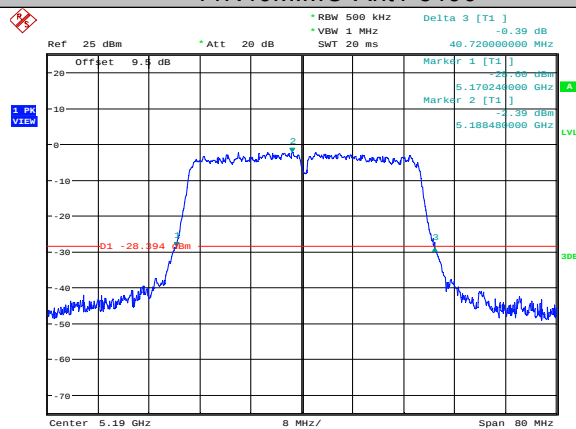
11N40MIMO-Ant1-5190
