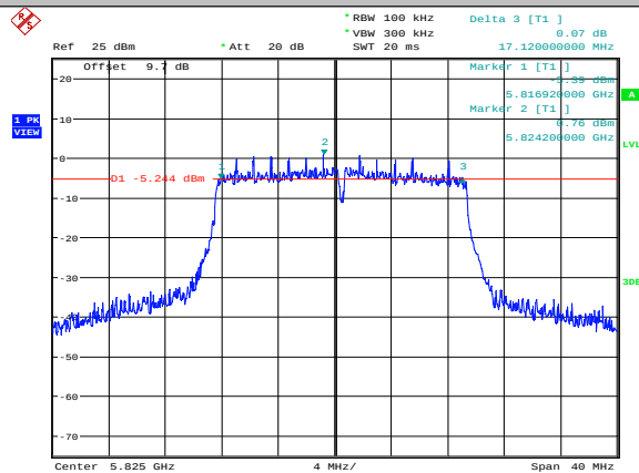
11N20MIMO-Ant1-5825
