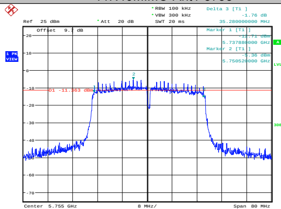
11N40MIMO-Ant1-5755
