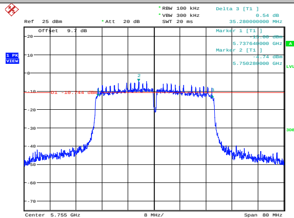
11AC40MIMO-Ant1-5755
