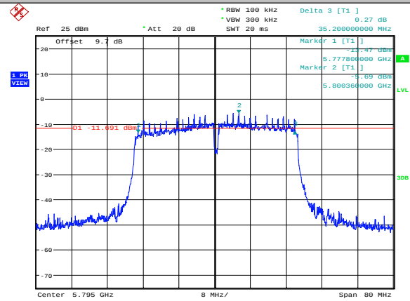
11N40MIMO-Ant2-5795
