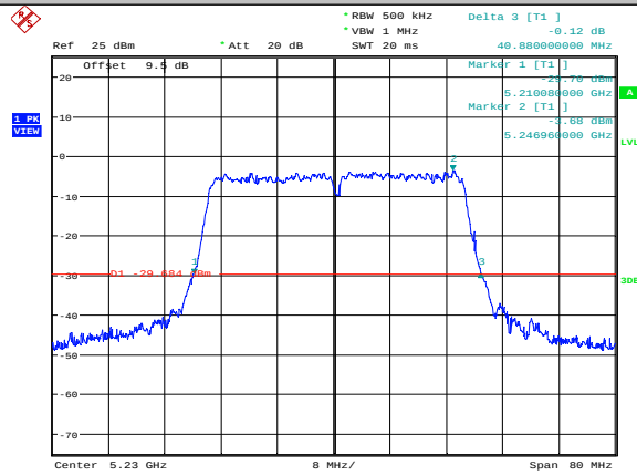
11N40MIMO-Ant1-5230
