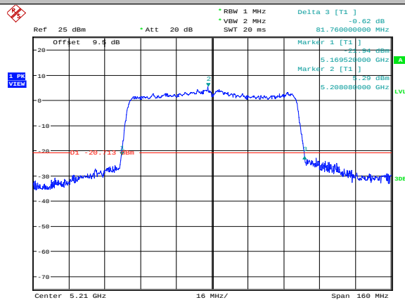
11AC80SISO-Ant1-5210
