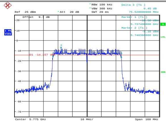
11AC80SISO-Ant2-5775
