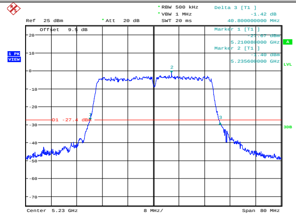
11N40MIMO-Ant2-5230
