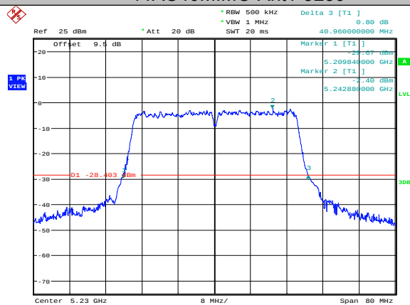
11AC40MIMO-Ant1-5230
