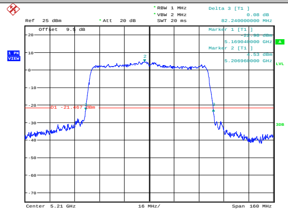
11AC80SISO-Ant2-5210
