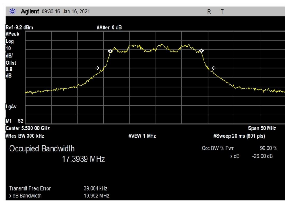
99%BW 802.11VHT20
