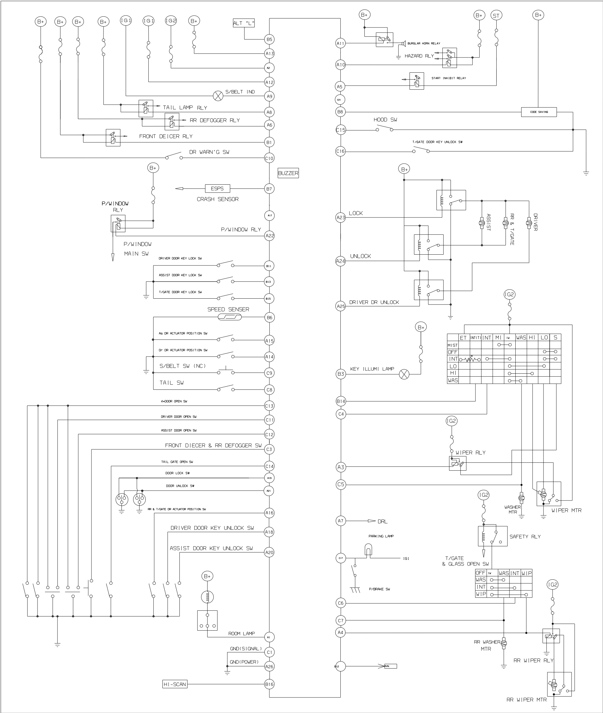
△△△△△ KEYLESS (복미 사양)
