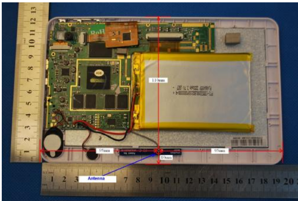
Fig.17-4 Antenna
