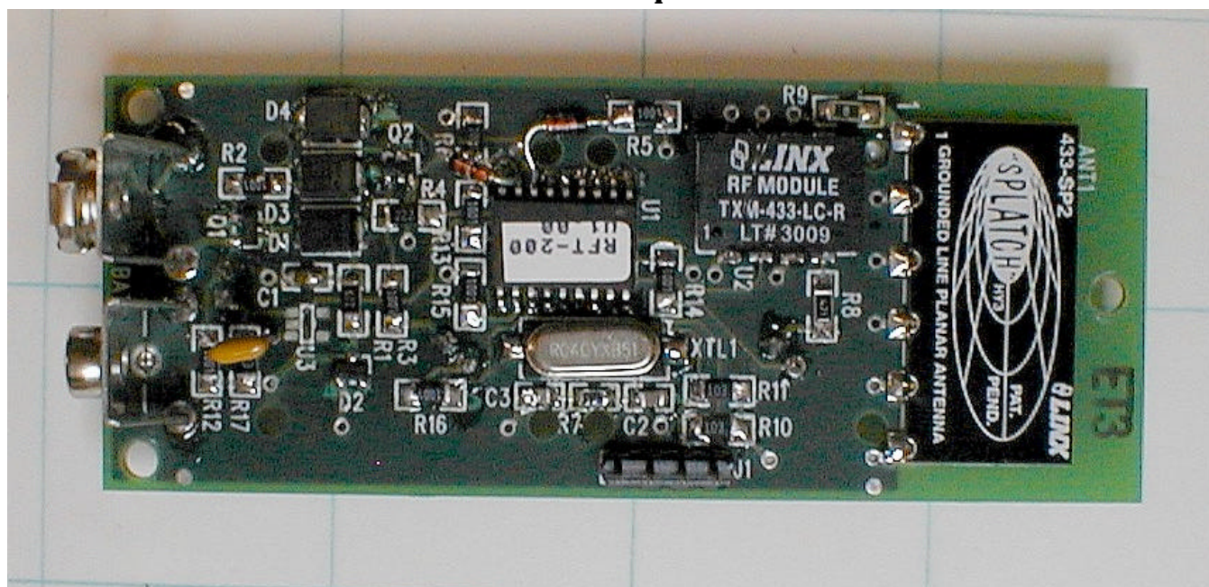
PCB Top
