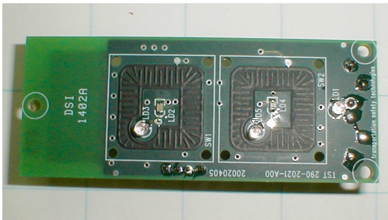
PCB Bottom
