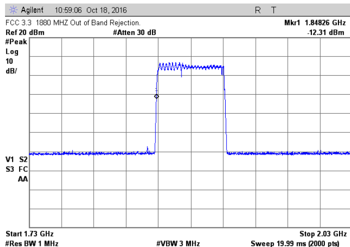
PCS 1850-1910 MHz
