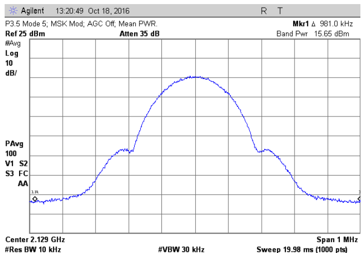
2129 MHz; MSK
