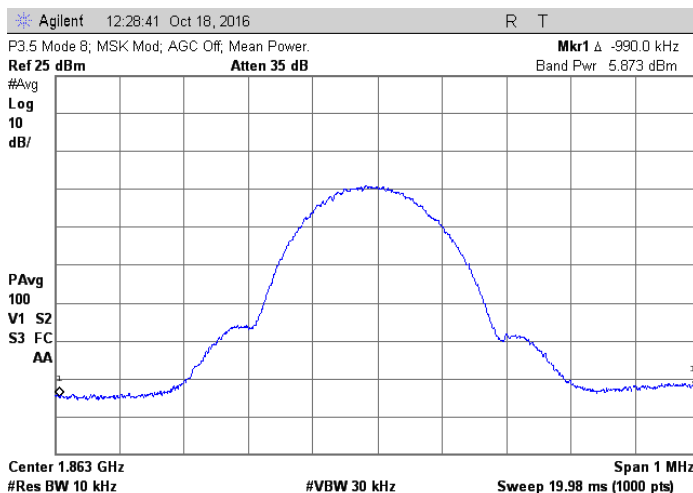
1863 MHz MSK
