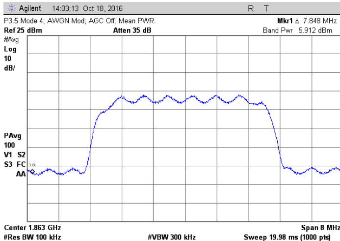
1863 MHz AWGN
