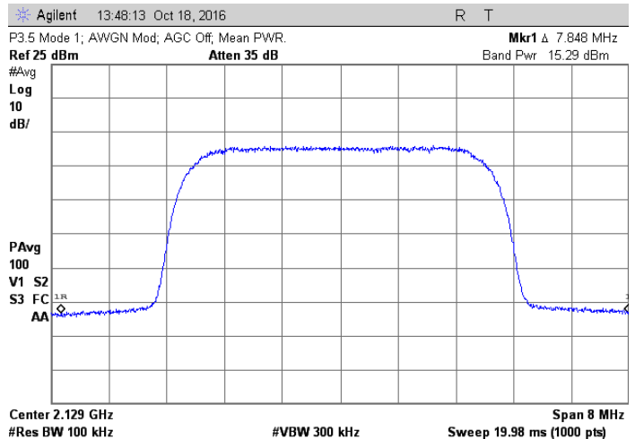
2129 MHz; AWGN
