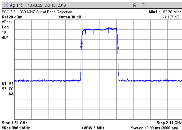
PCS 1930-1990 MHz
