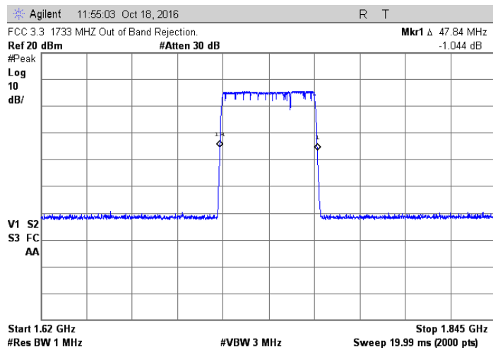
AWS 1710-1755 MHz
