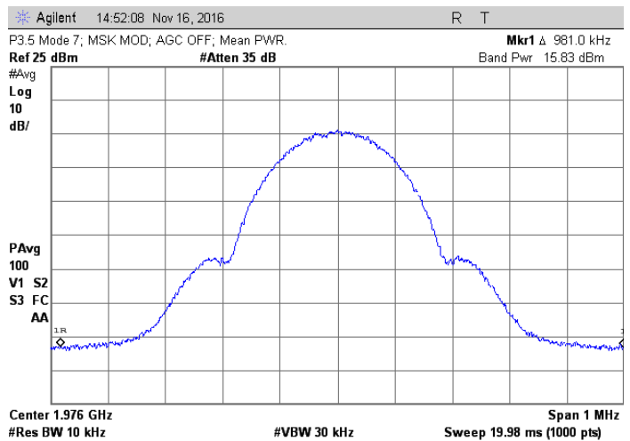
1976.2 MHz; MSK
