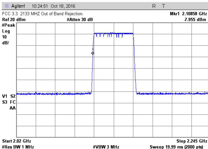
AWS 2110-2155 MHz
