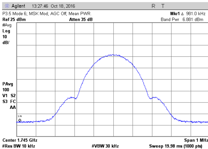
1745 MHz MSK
