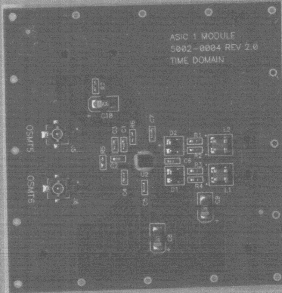
ASIC 1 Module Top
