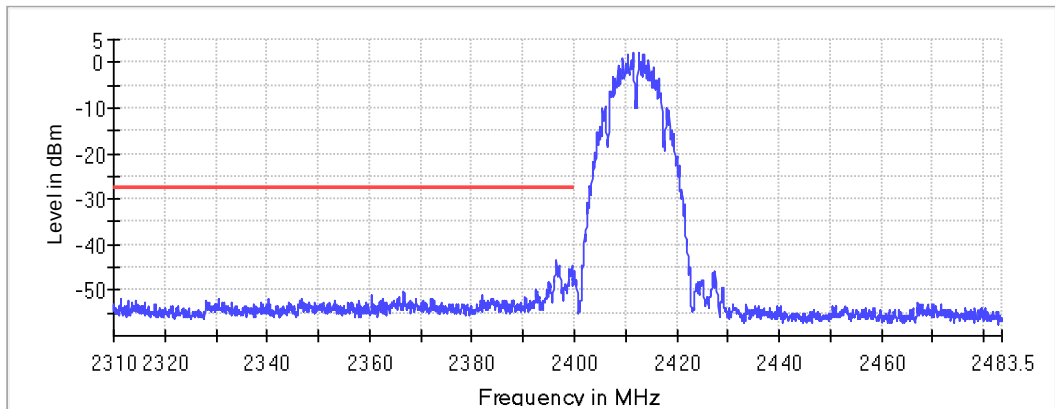
Band Edge
