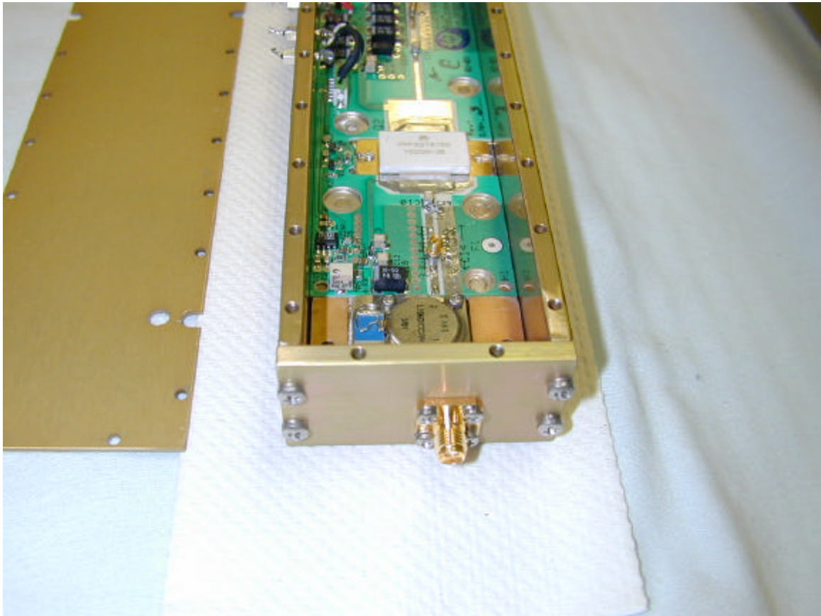
Amplifier Module (Output End)
