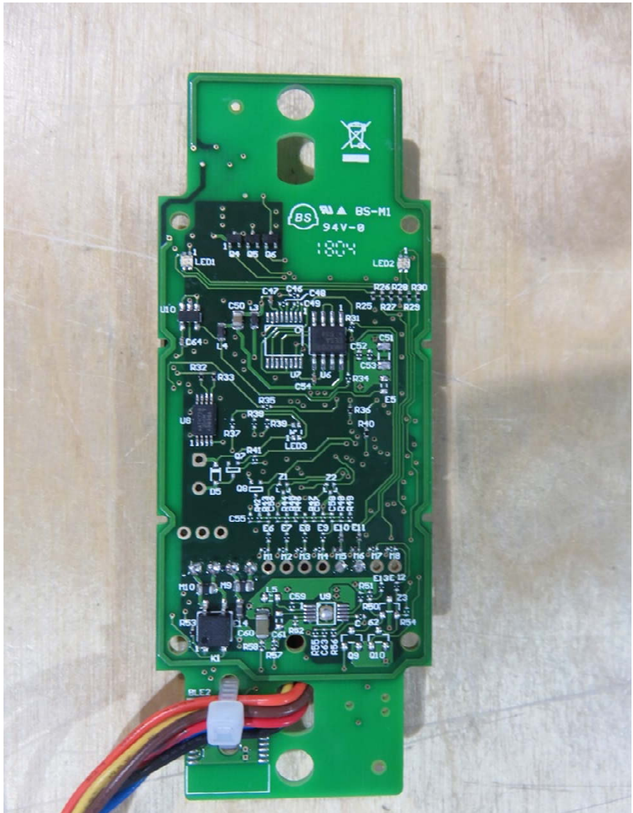
EUT BOTTOM
