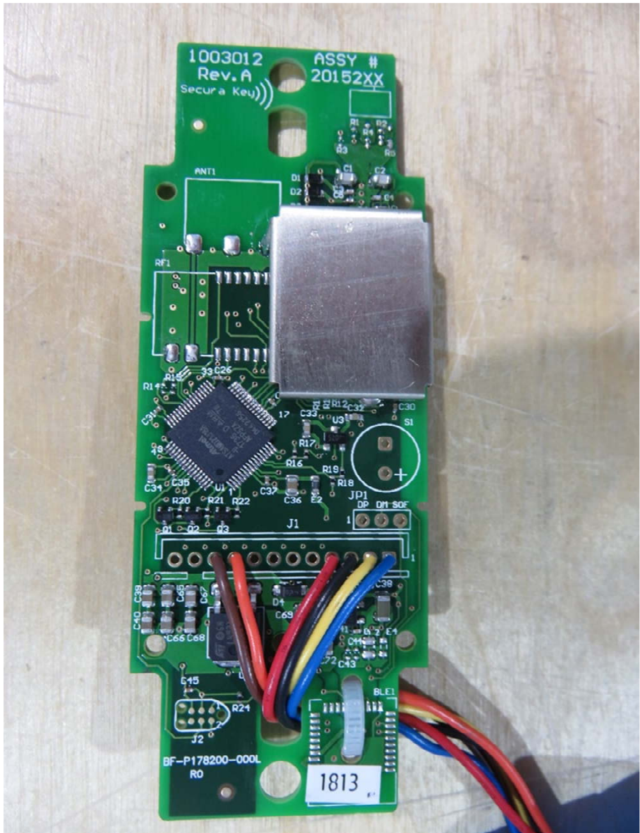
EUT TOP
