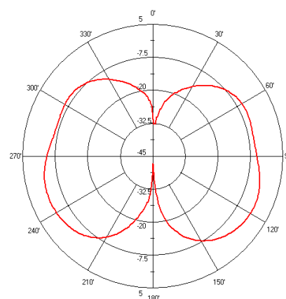
AN9520 E-Plane
