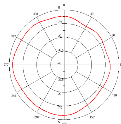
AN9520 E-Plane
