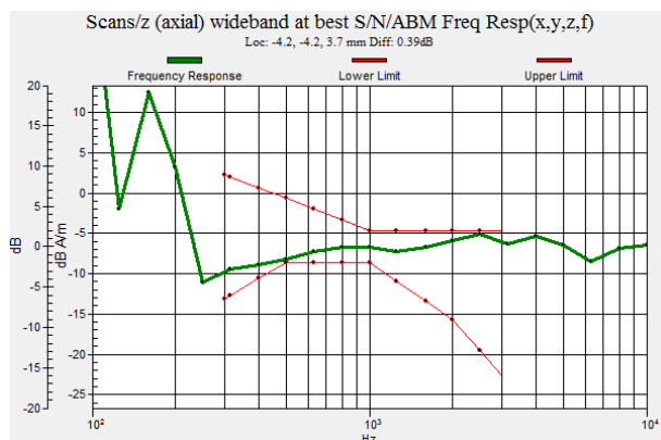
Fig. 9.9 CDMA2000 BC15 Ch25
