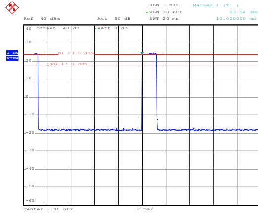
1900MHz - CDMA (1/8 Rate)
