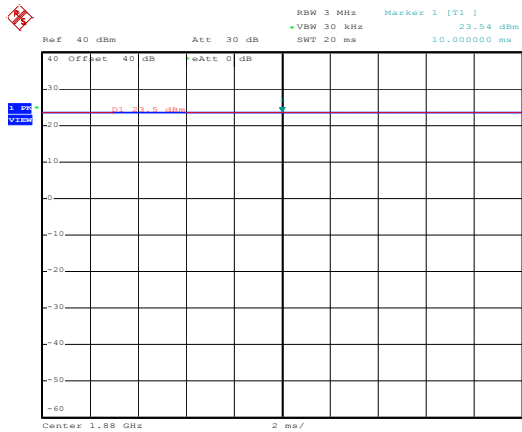
1900MHz - CW
