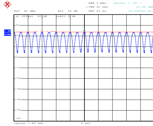
1900MHz - 80% AM
