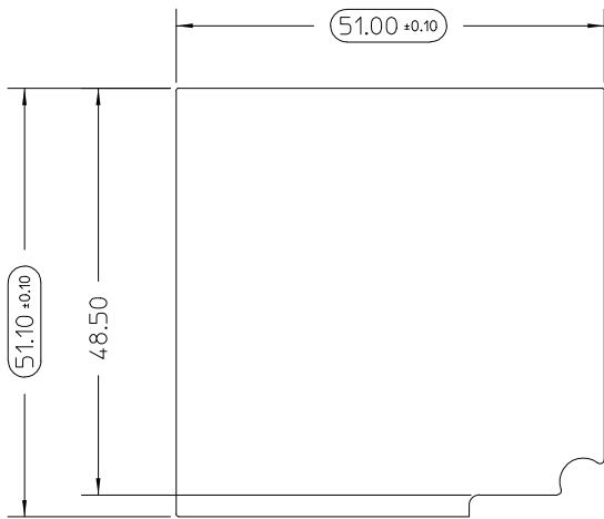
Front1
