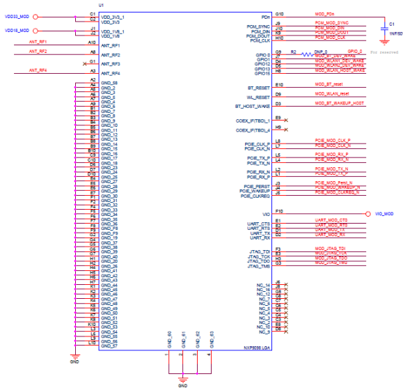
88Q9098 Module
