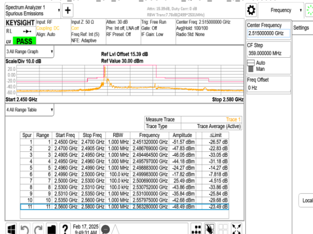
Band7_30MHz_CP_OFDM_SCS15kHz_QPSK_RB1_159_CH503000
