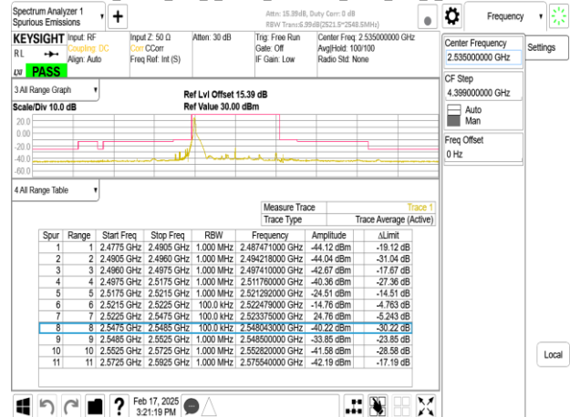
Band7_25MHz_DFT_s_OFDM_SCS30kHz_BPSK_RB1_64_CH507000
