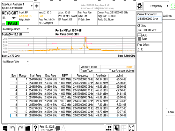
Band7_30MHz_CP_OFDM_SCS15kHz_QPSK_RB1_159_CH507000
