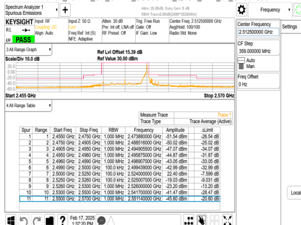
Band7_25MHz_CP_OFDM_SCS30kHz_QPSK_RB65_0_CH502500
