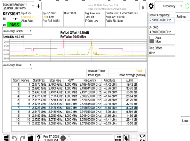
Band7_25MHz_CP_OFDM_SCS30kHz_QPSK_RB65_0_CH507000
