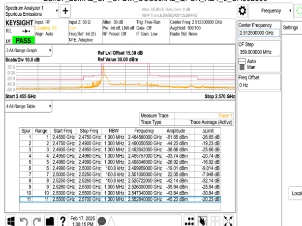
Band7_25MHz_CP_OFDM_SCS30kHz_QPSK_RB1_64_CH502500
