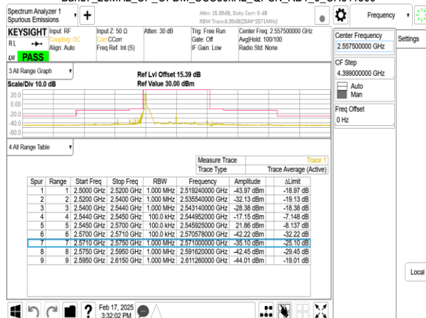
Band7_25MHz_CP_OFDM_SCS30kHz_QPSK_RB1_64_CH511500
