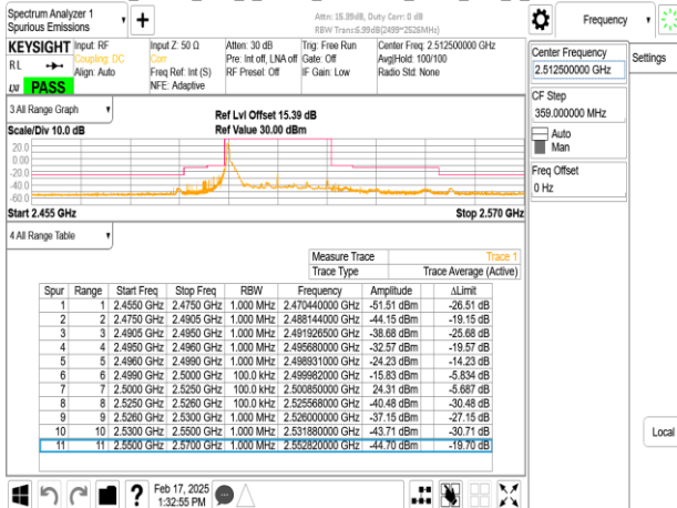
Band7_25MHz_DFT_s_OFDM_SCS30kHz_BPSK_RB1_64_CH502500
