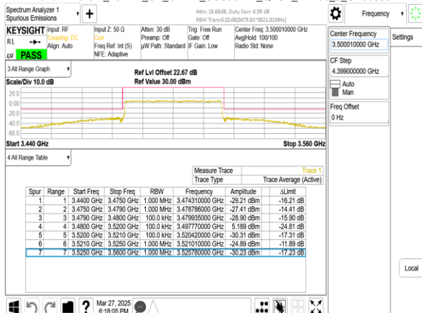
Band77-Part27_40MHz_CP_OFDM_SCS30kHz_QPSK_RB1_0_CH633334
