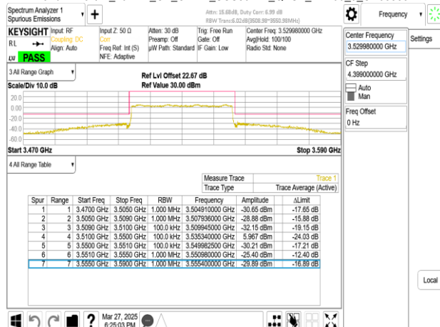
Band77-Part27_40MHz_CP_OFDM_SCS30kHz_QPSK_RB1_0_CH635332
