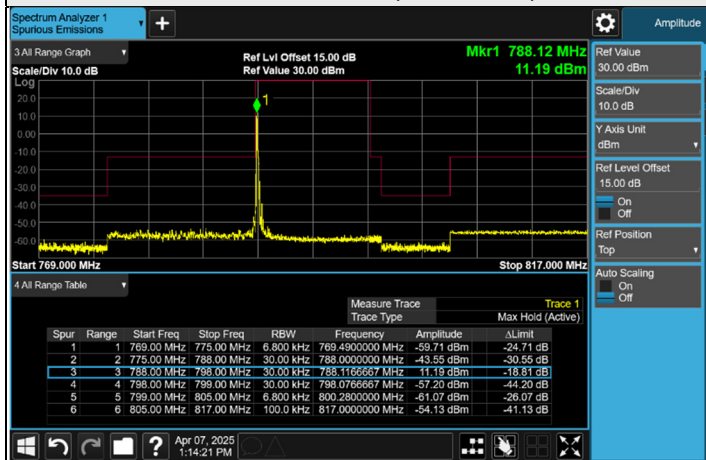
1RB CH 23282 (788.2 MHz)
