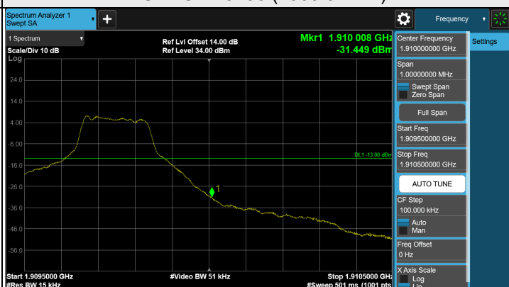
1RB CH 19193 (1909.3 MHz)
