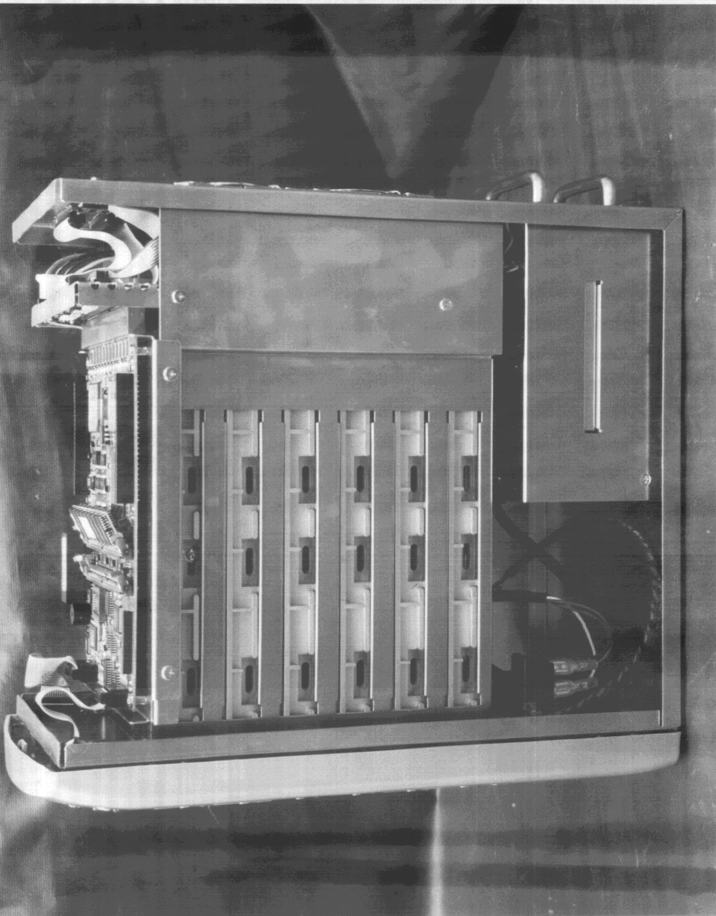
FCC ID : NKE-SILVER PHOTO 3. EUT INSIDE VIEW
